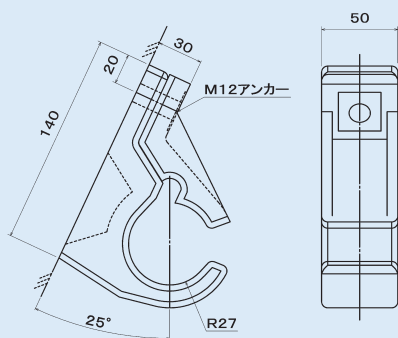
FRP-LCX支持具
