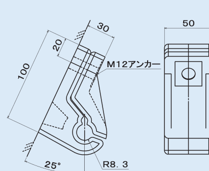
FRP-SLCX 支持具 (D12)
