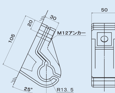
FRP-SLCX 支持具 (D16)
