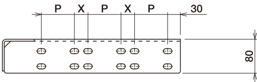
ソフトUボルトベース 4条用 (LQ)
