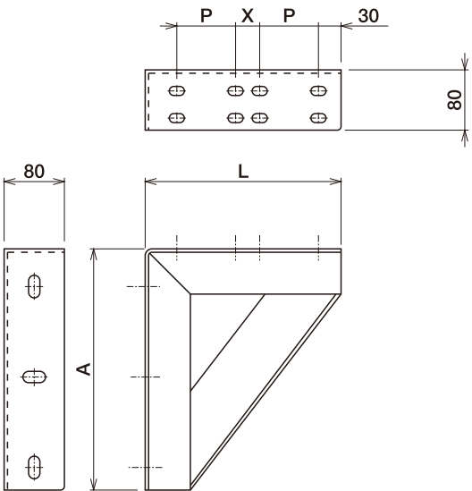
ソフトUボルトベース 2条用 (DW)
