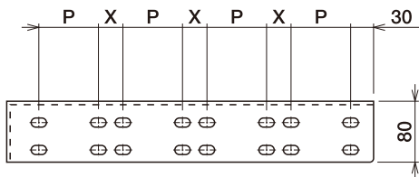
ソフトUボルトベース 4条用 (DQ)
