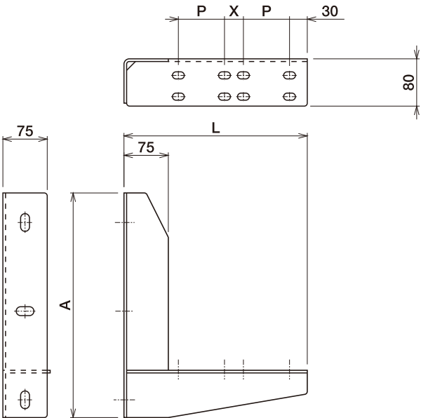
ソフトUボルトベース 3条用 (LT)
