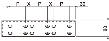
ソフトUボルトベース 4条用 (DQ)
